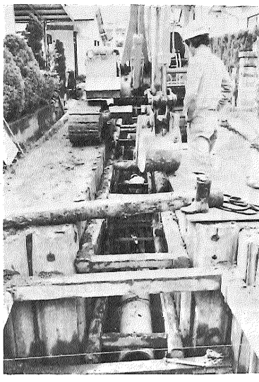
伸びゆく下水道、汚水管の埋設工事(鬼丸町)
