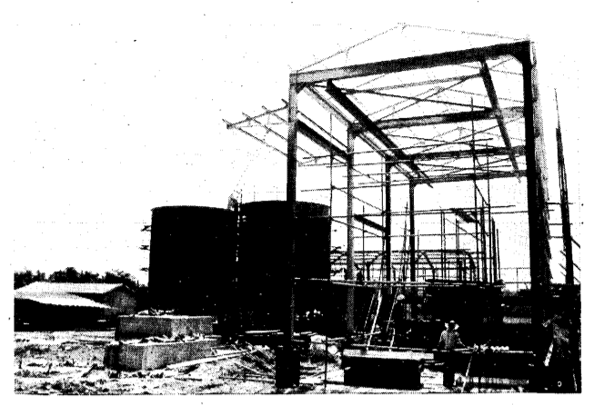
フジコンポストシステムの建設すむ現場
