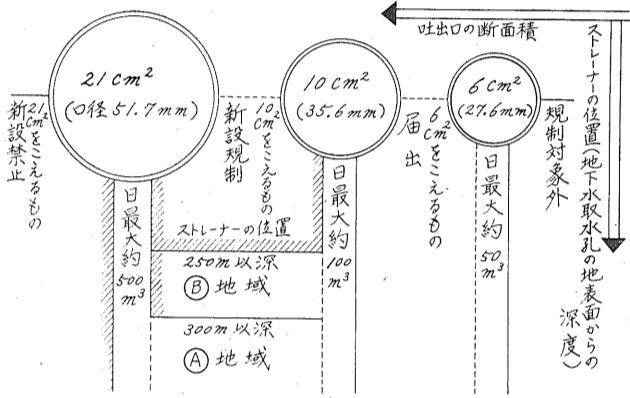
地下水採取規制概要略図
