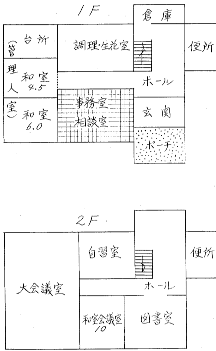
教育集会所平面図
