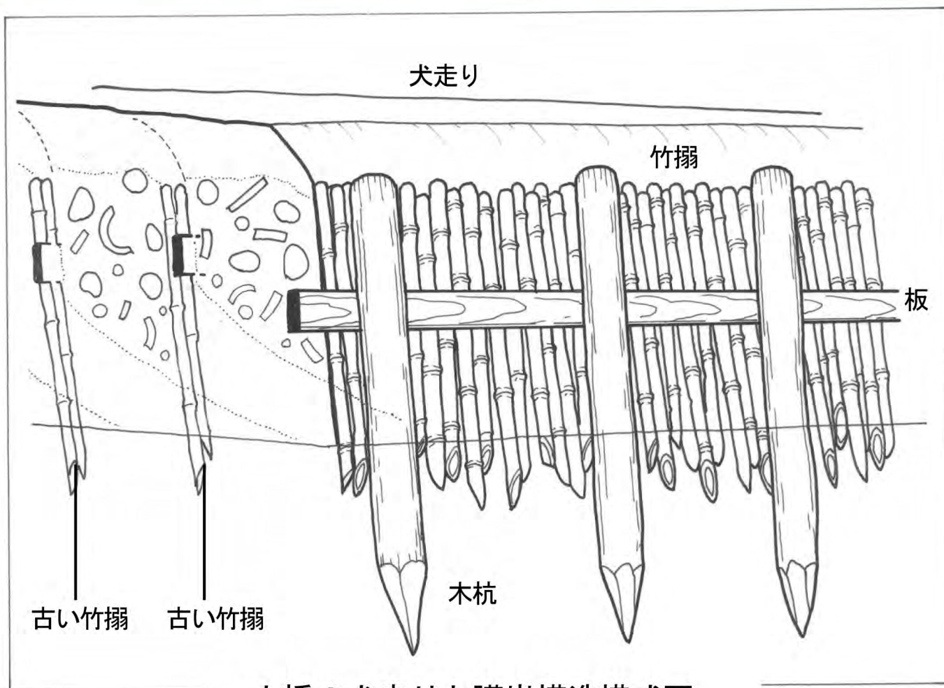
土橋の犬走りと護岸構造模式図
