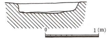
Fig. 4 S K002土壇実測図 (S = 1/40)
