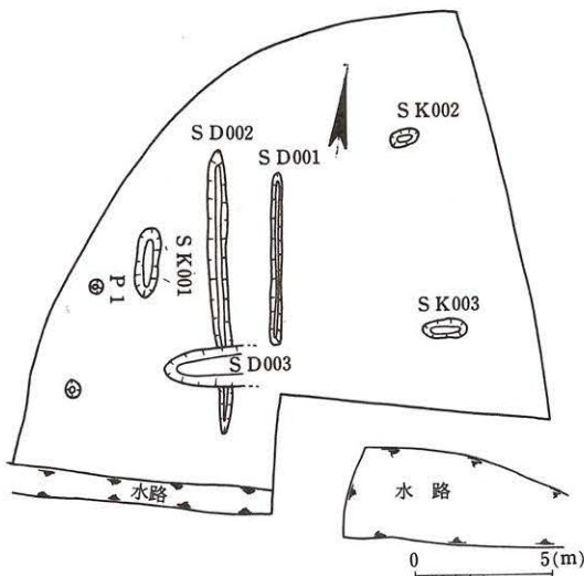
Fig. 9 開成小学校内遺跡遺構配置図 (1/200)
