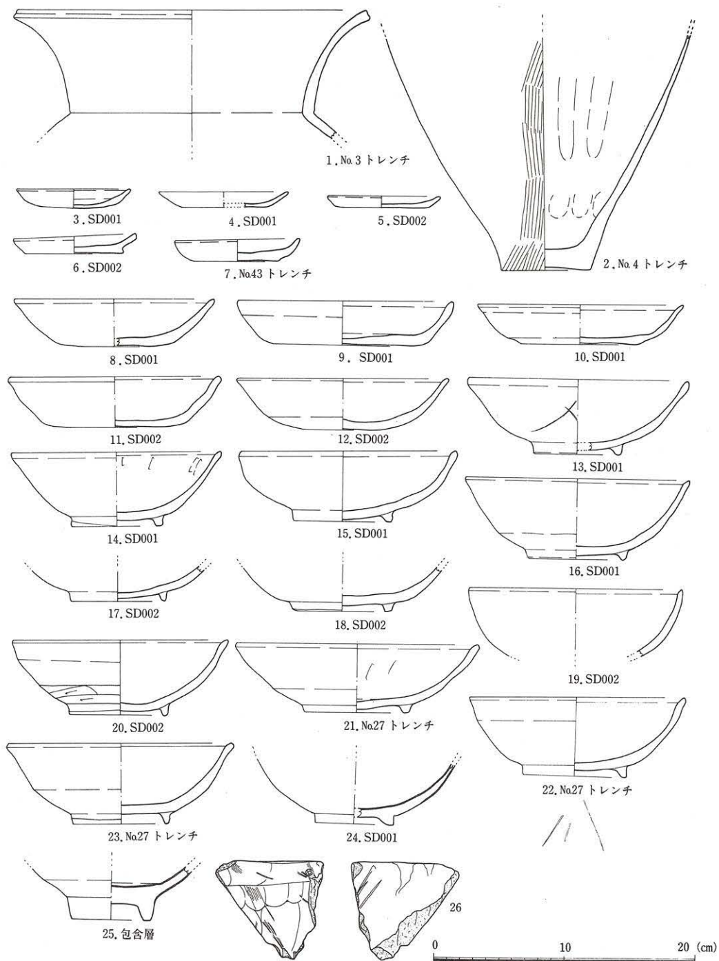
Fig. 7 開成小学校内出土遺物実測図 (S = 1/4)
