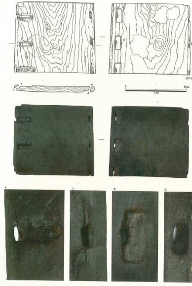
Fig. 010 関船解体材 (1/10)
