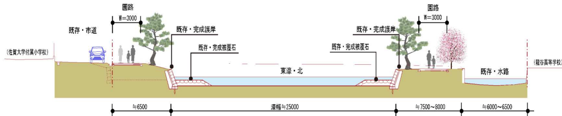
A-A'断面
