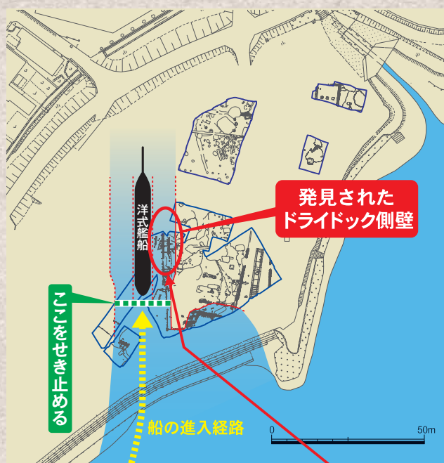
【ドライドック平面模式図】
