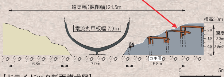
【ドライドック断面模式図】
