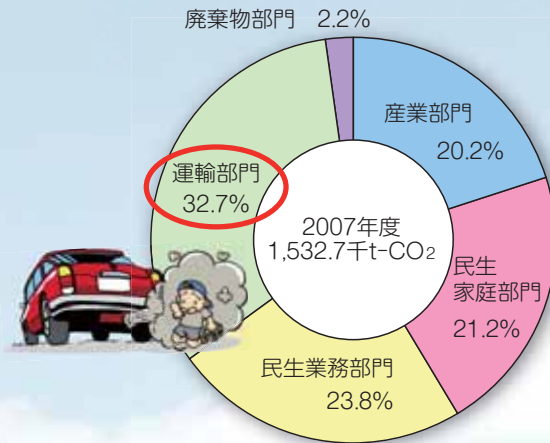
佐賀市における温室効果ガス排出量の部門別内訳
