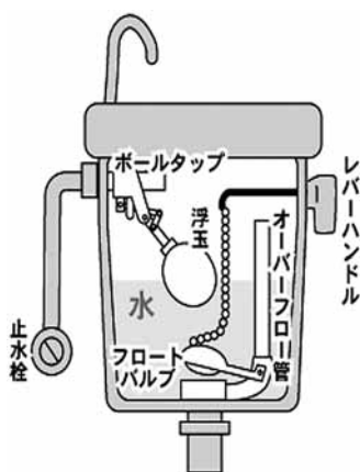
▲水洗トイレのタンクのしくみ
