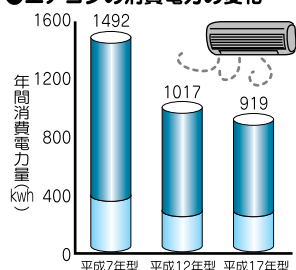
●エアコンの消費電力の変化
