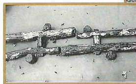
▲ 石垣の下部には沈下を防ぐため「はしご状胴木」を用いている
