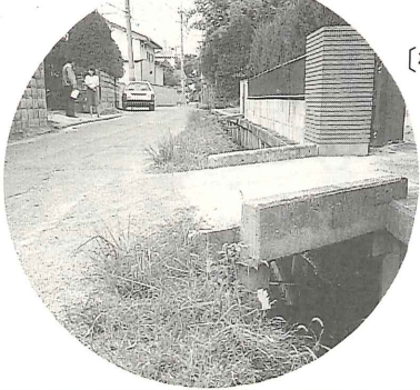
〔間知ブロック〕 より強い護岸
