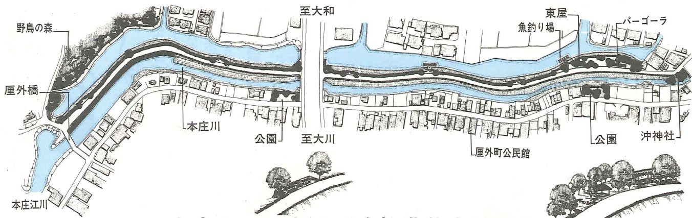
末広1丁目水辺環境整備基本計画図
