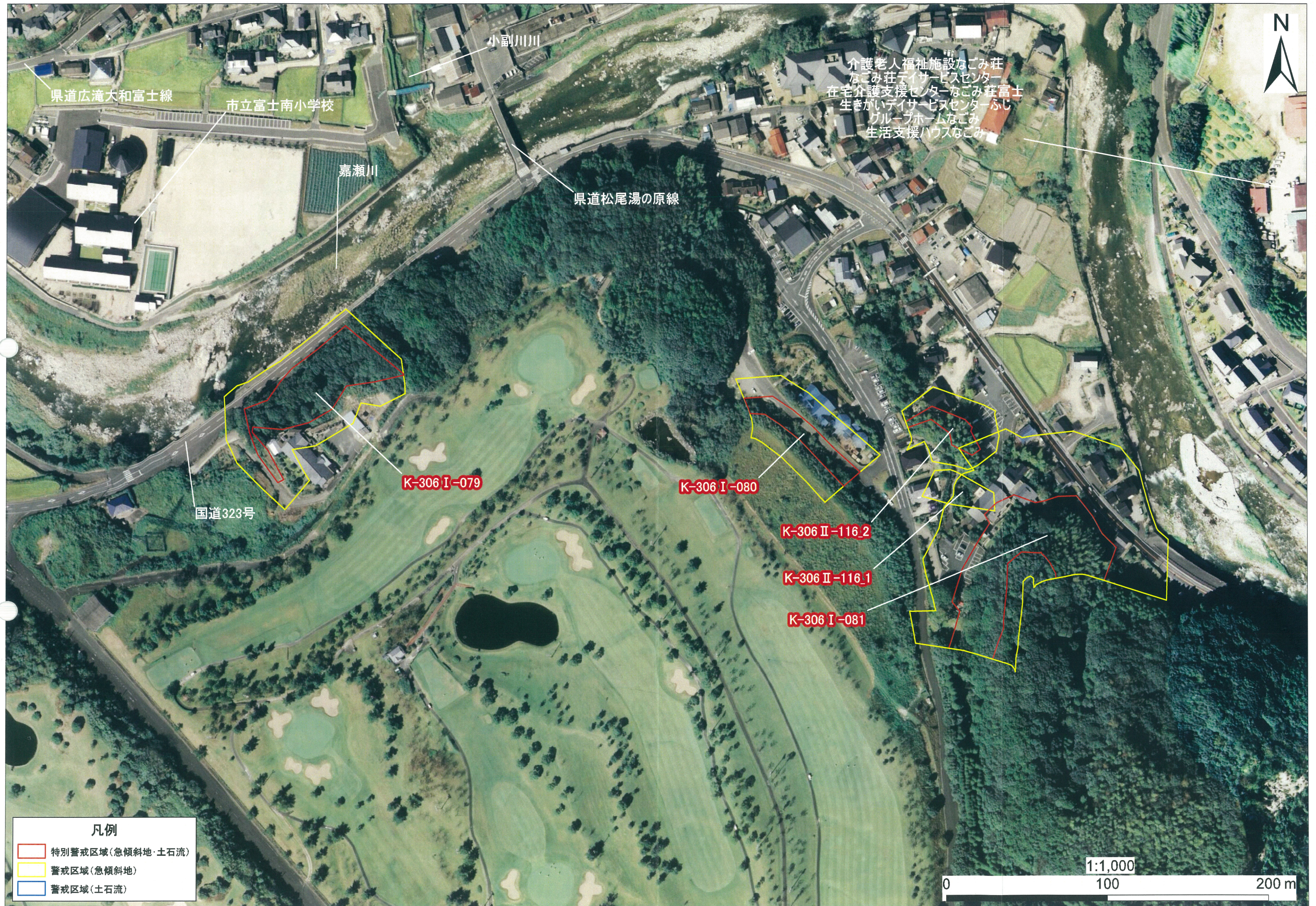
土砂災害警戒区域図-7(上熊川地区⑦)
