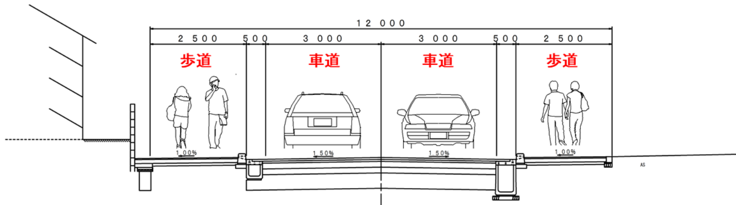
標準断面図(一般区間)
