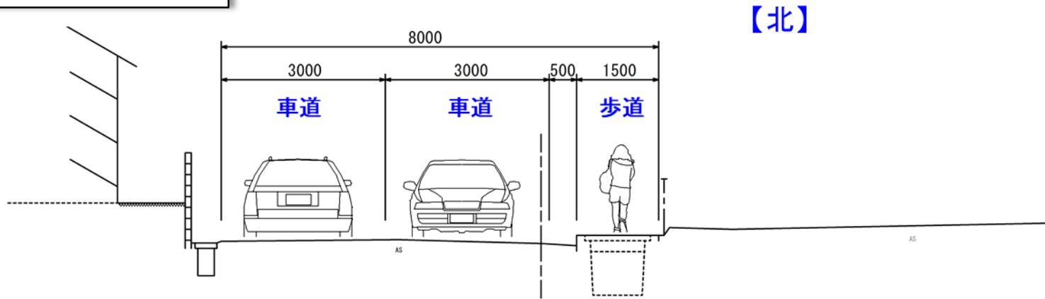
現況断面図(一般区間)
