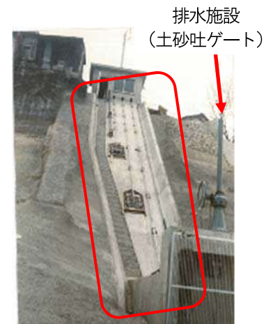
写真3：取水部（斜樋）
