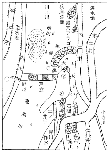
嘉瀬川石井樋平面図
