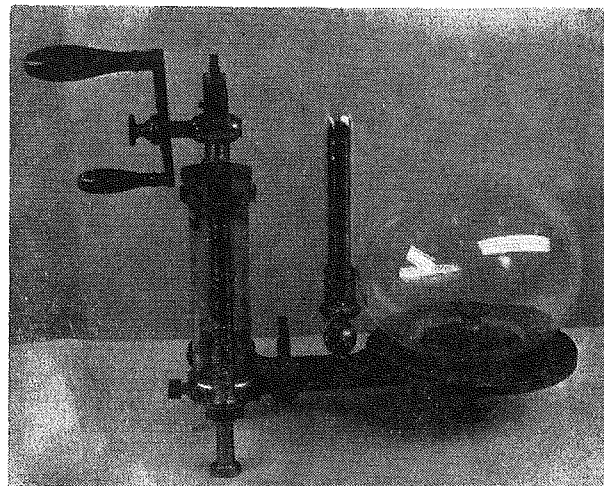
精煉方の道具・真空ポンプ（佐賀県立博物館蔵）
